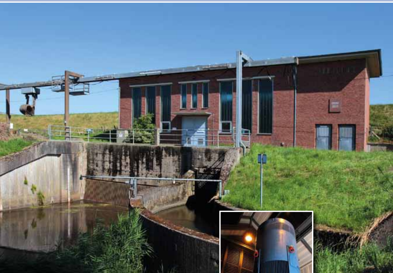
Das Schöpfwerk St. Annen mit zwei unterschiedlich einzuhaltenden Wasserständen (gr. Bild). Zum Innenleben eines Schöpfwerks gehören auch die riesigen Pumpanlagen.
